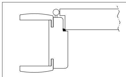
Coprifilo stondato mm 70 (su richiesta)
