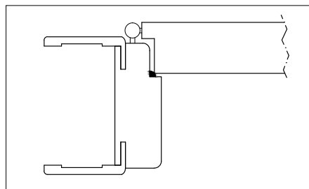
Coprifilo piatto mm 70 (di serie)
